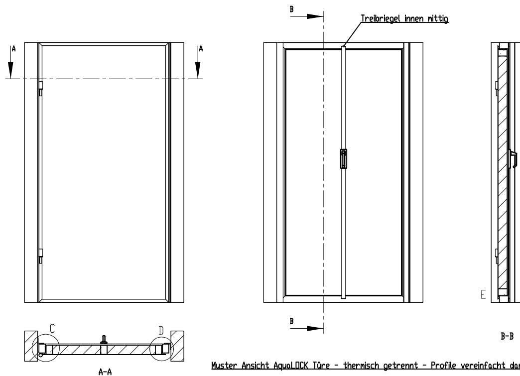
Muster Ansicht AquaLOCK Türe - thermisch getrennt - Profile vereinfacht dargestellt
