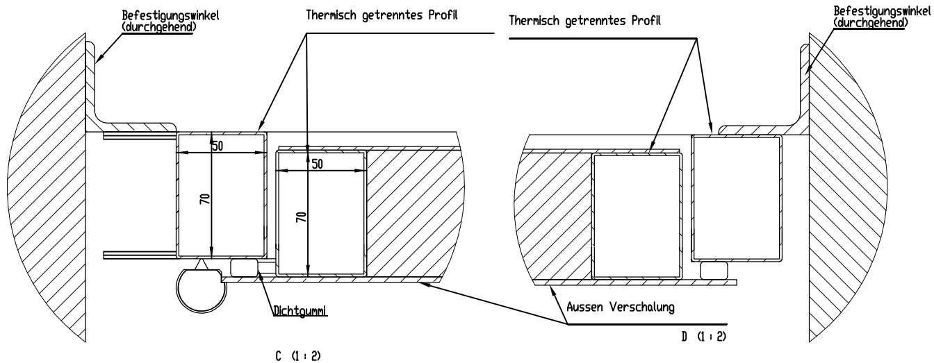
Muster Ansicht AquaLOCK Türe - thermisch getrennt - Profile vereinfacht dargestellt
